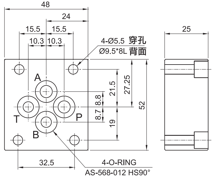
安裝面 Mounting Interface: ISO 4401-AB-03-4-A
